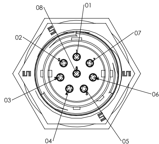
-03: 8 POS ( \varnothing 1.5 SOCKETS)
