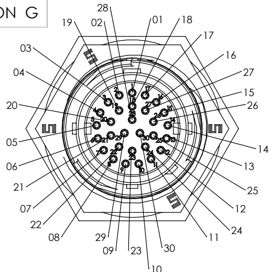
-01: 30 POS ( \varnothing 1.0 SOCKETS)
