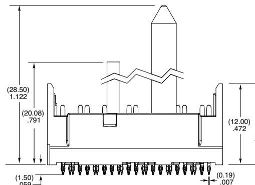
HDTM-6-04-X-X-VT-4-L-X-A SHOWN
